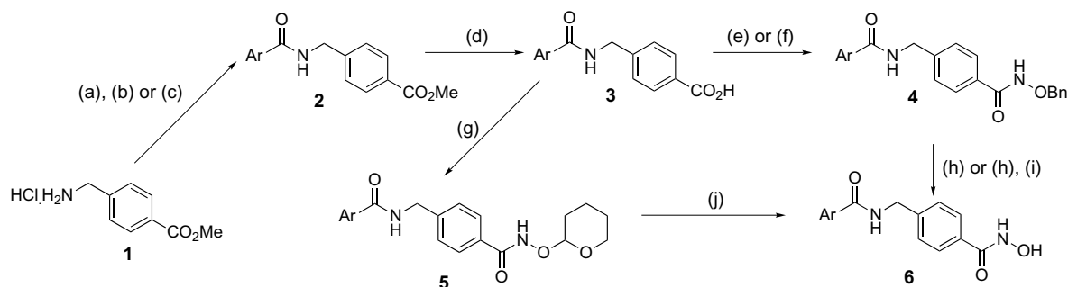
Scheme 1. Conditions: (a) ArCOCl, Et 3 N/CH 2 Cl 2 ; (b) ArCO 2 H, BOP-Cl, Et 3 N/DMF; (c) ArCO 2 H, HONB, WSCI, Et 3 N/DMF; (d) 1 M LiOH/H 2 O–THF; (e) H 2 N–OBn, BOP-Cl, Et 3 N/CH 2 Cl 2 or DMF; (f) H 2 N–OBn, HONB, WSCI, Et 3 N/DMF; (g) NH 2 OTHP, HONB, WSCI, Et 3 N/CH 2 Cl 2 –DMF; (h) H 2 /5% Pd–C/MeOH or H 2 /10% Pd–C/MeOH; (i) 12 N HCl/MeOH; (j) CH 3 CO 2 H–THF–H 2 O.
